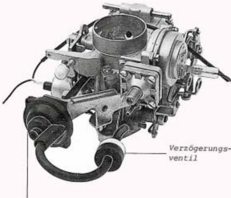
Schließdämpfer
